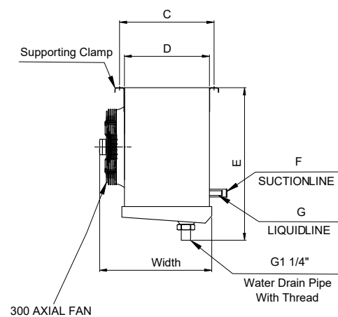
300 AXIAL FAN
