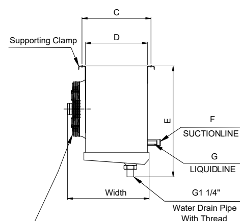
300 AXIAL FAN
