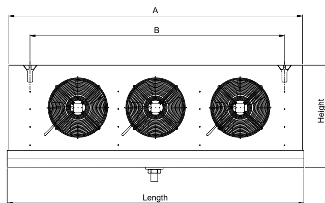
300 AXIAL FAN
