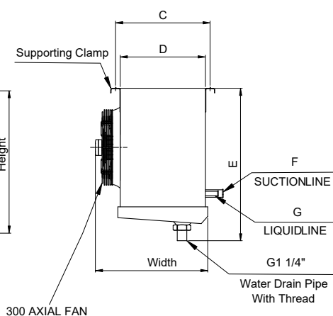
300 AXIAL FAN
